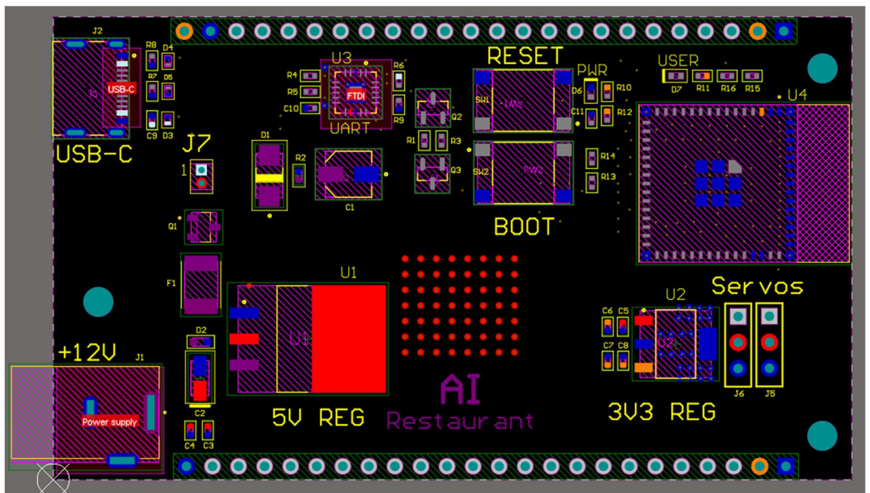
Vizualizarea stratului de componente
