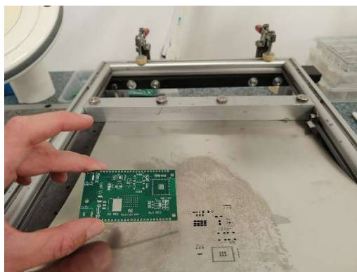
Aplicarea pastei de lipit pe PCB
