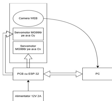
Figura 4.1 - Schema bloc
