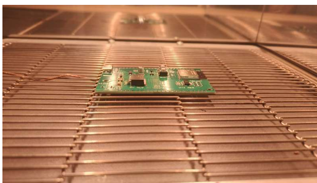
Reflow în cuptorul cu convecție
