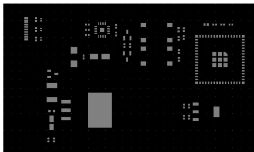
Strat de pastă – parte superioară
