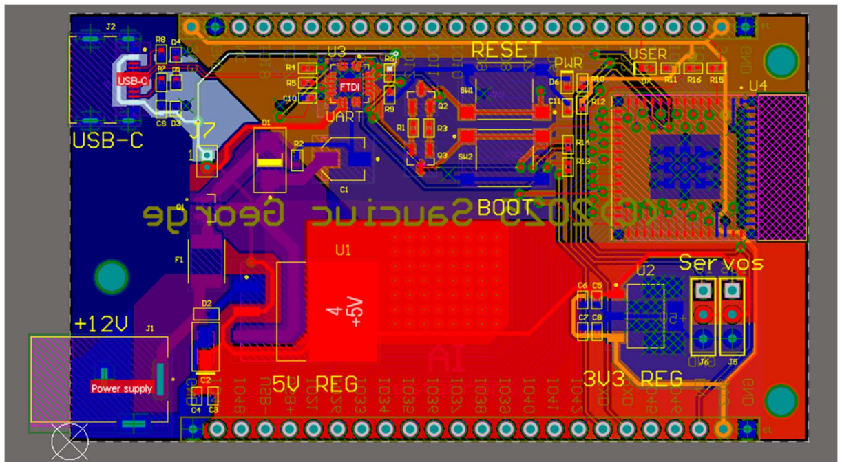
Vizualizarea completă a plăcii PCB
