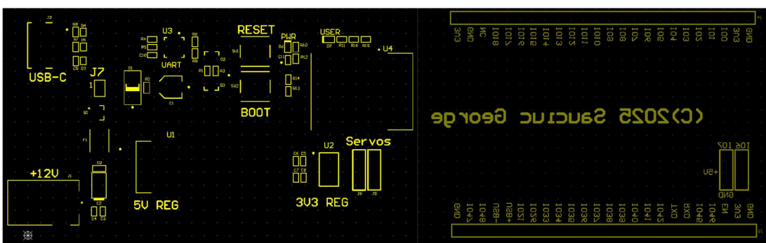
Strat de serigrafie – parte superioară
