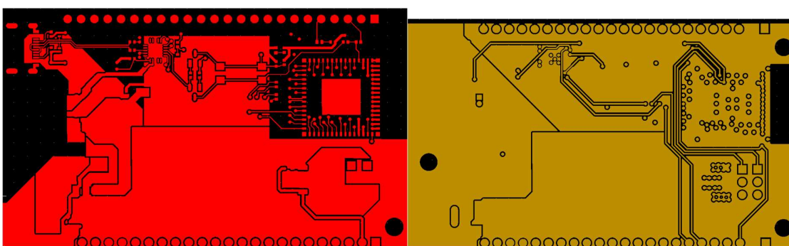
Strat de semnal – parte superioară
