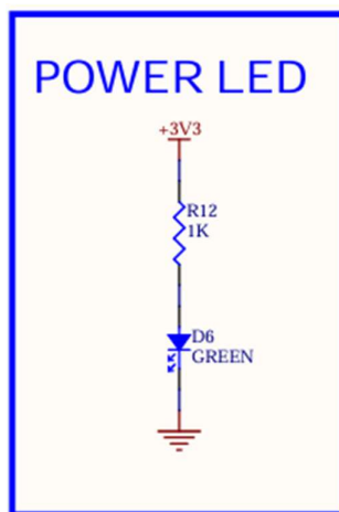
Figura 4.22 - LED-ul Power
