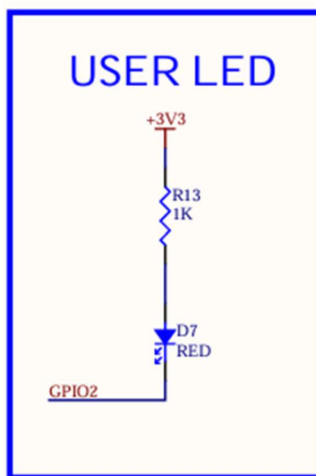
Figura 4.23 - LED-ul User
