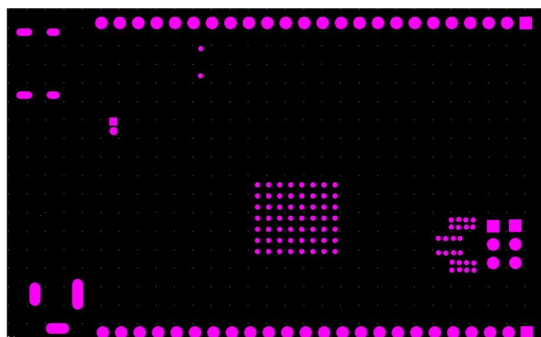
Strat de mască de lipire – parte inferioară
